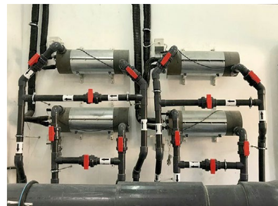
Čtyři tepelné výměníky HP 3000 v provedení SPLIT, Dubaj (140 kW)
