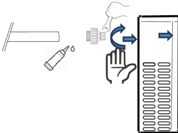
Ábra: Külső menettel rendelkező tömlő PN16. G=6/4" D=50mm
