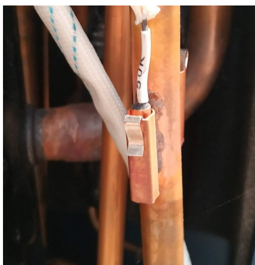
T4 – Kompresszor kisülési hőmérséklete
