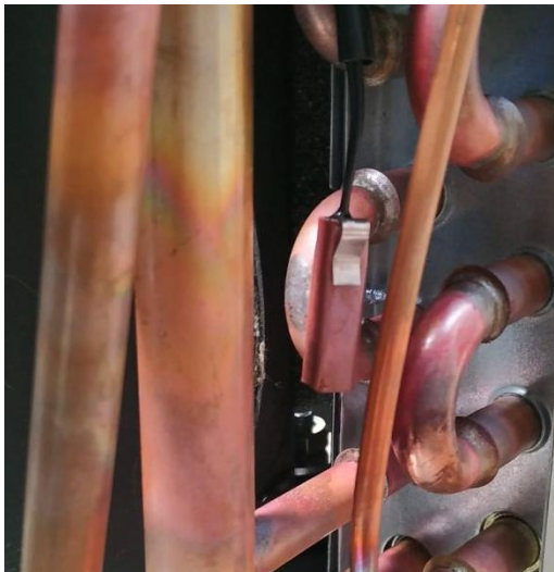
T3 – Környezeti levegő hőmérséklet
