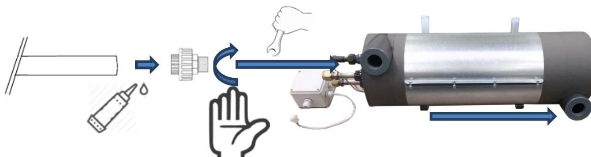
Obrázok: Vzorové pripojenie vody na tepelné čerpadlo. Pružná hadica je nalepená na adaptér matice hadice s vonkajším závitom, ktoré je upevnené na závit výmenníka tepelného čerpadla.
