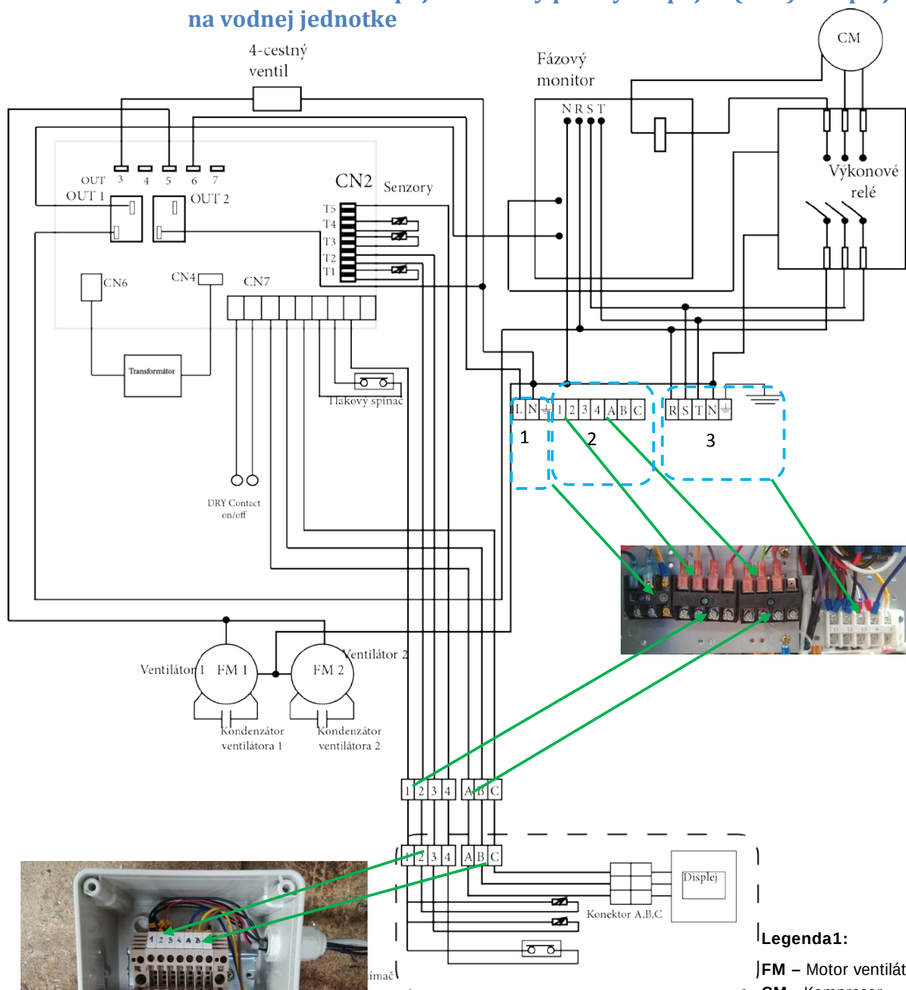
T2, T5, prietokový spínač a pripojenie dosky displeja na vodnej jednotke
