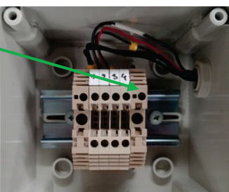
T2, T5, pripojenie spínača prietoku na vodnej
