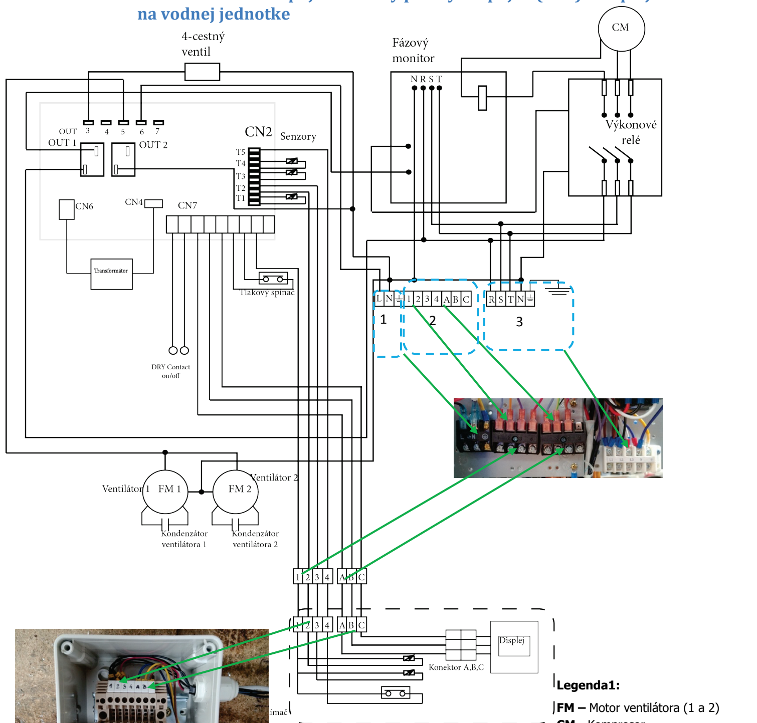
T2, T5, prietokový spínač a pripojenie dosky displeja na vodnej jednotke
