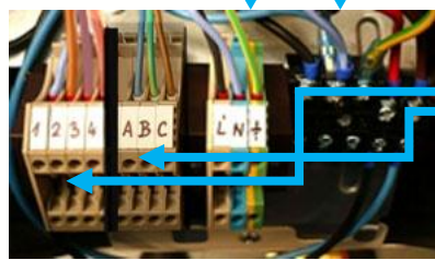
Obrázok: Zdroj napätia tepelného čerpadla a prídavného obehového čerpadla a senzory 1-4 vodnej jednotky (hore) a A,B,C konektor pre displej.
