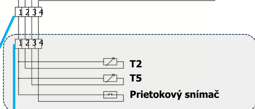
Obrázok: Pripojenie zdroja napätia tep. čerpadla vzduchovej jedn. a prídavného obehového čerpadla a senzorov 1-4 vodnej jednotky.
